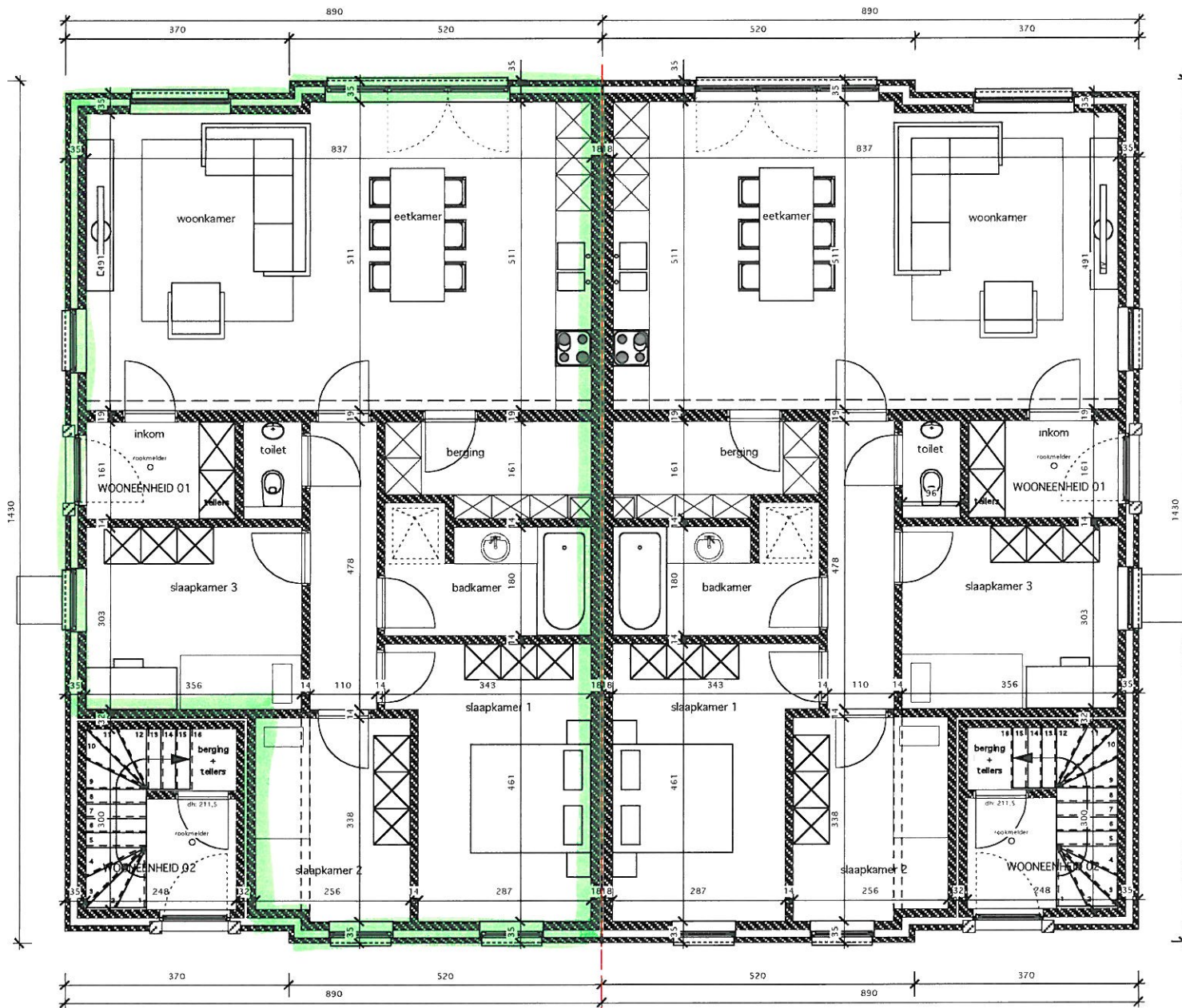
GELIJKVLOERS schaal 1/100
