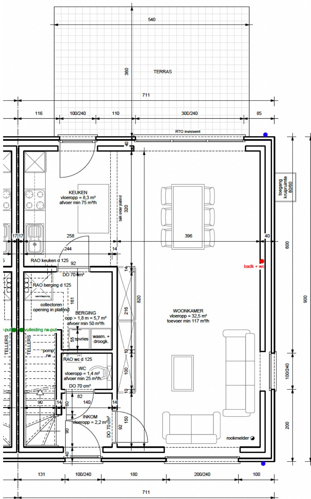
Grondplan
