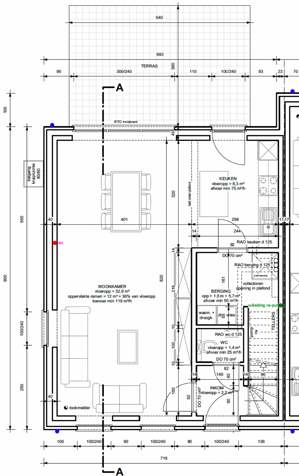
Grondplan
